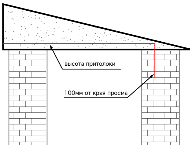
Рис. 10 Места крепления ворот к стенам. Вид на правый заплечик изнутри проема
