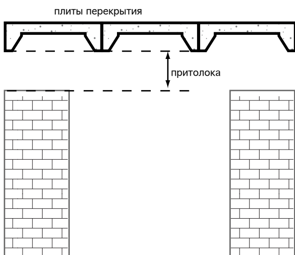
Рис. 12 Потолок из плит с ребрами жесткости
